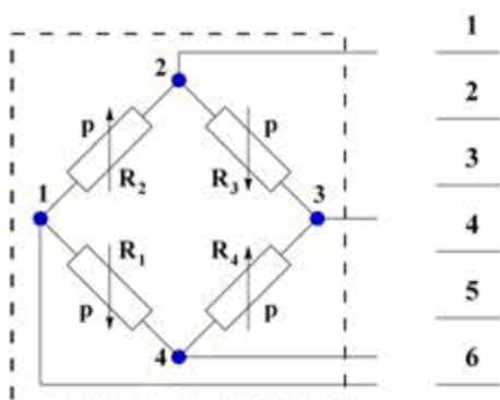
Схема подключения
