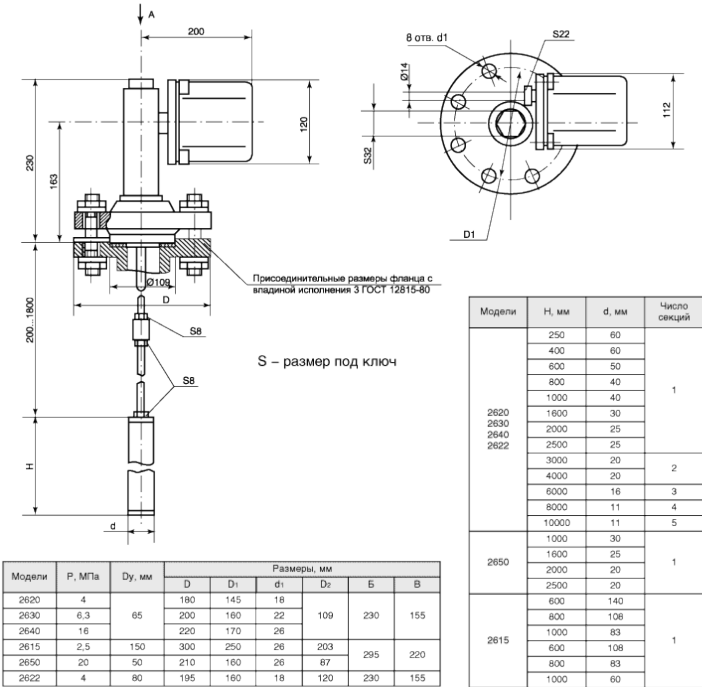
Рис. 1. Общий вид, габаритные, установочные и присоединительные размеры преобразователей УБ-ЭМ
