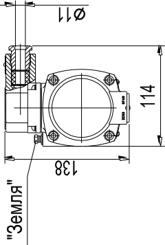
Рисунок 3. Для моделей по табл. И.8
