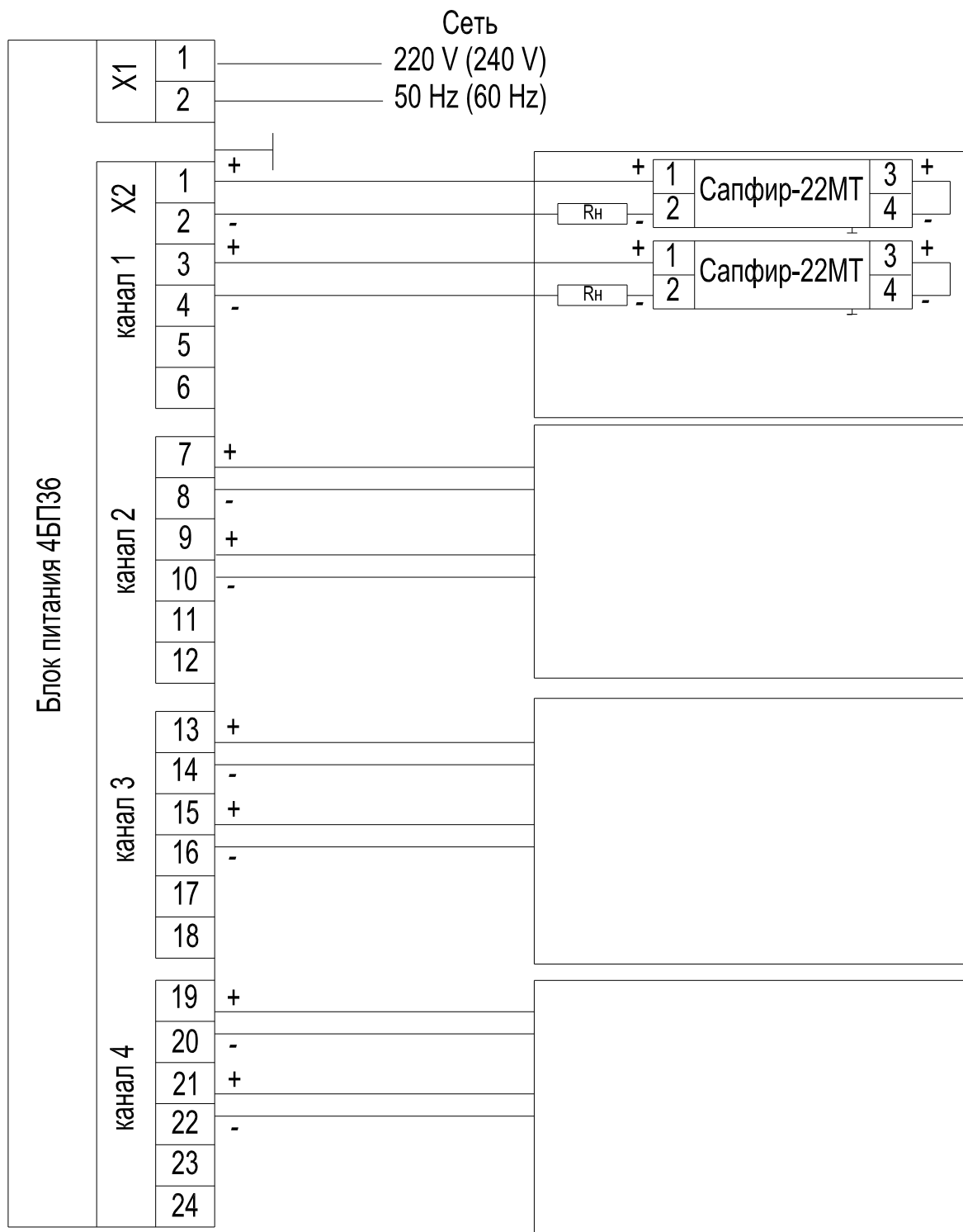
Схема электрическая подключения преобразователя Сапфир-22МТ и блока питания 4БПЗ6 по двухпроводной схеме
