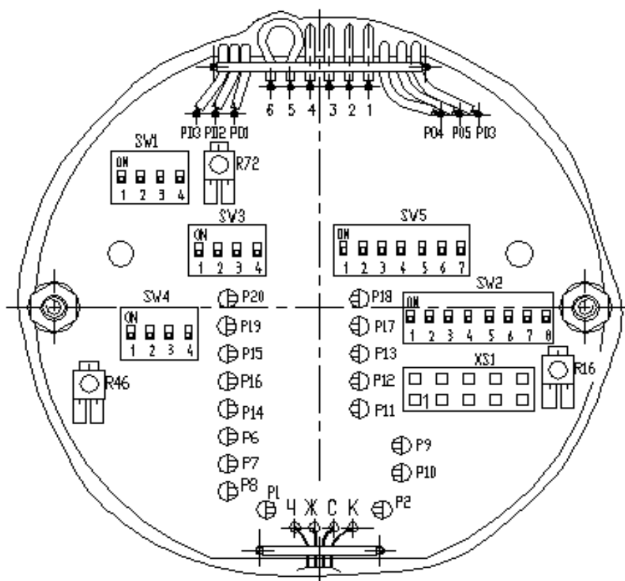
Рисунок 1 Внешний вид платы с элементами регулировки
